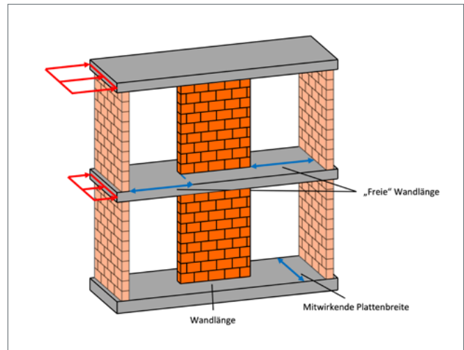
Abbildung 7.4: Darstellung der Eingabeparameter am Beispiel einer zweigeschossigen Schubwand mit Querwänden [14]
